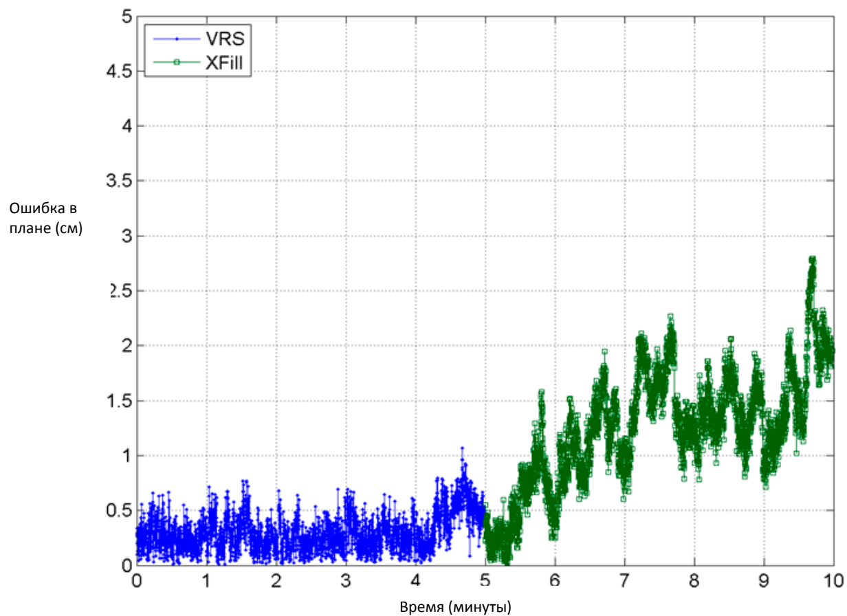
Рисунок 10. Ошибка определения координат в плане при работе в режиме Trimble xFill
