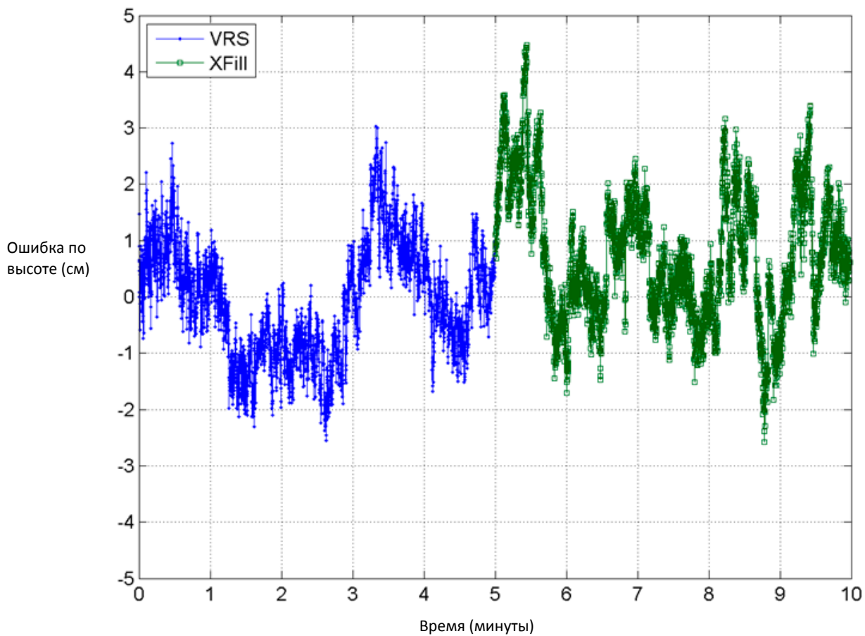
Рисунок 11. Ошибка определения координат по высоте при работе в режиме Trimble xFill
