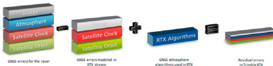
Рисунок 8. Моделирование ошибок в Trimble RTX
