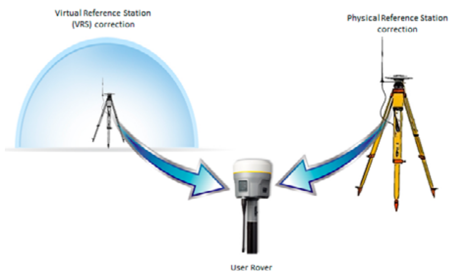
Рисунок 3. Возможные источники поправок для большинства RTK систем: одиночная физическая базовая станция или VRS сеть
