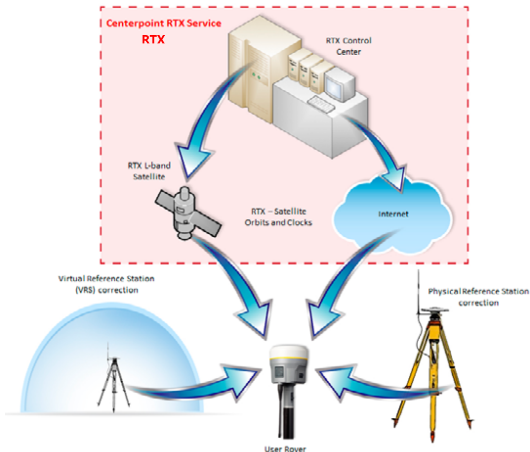
Рисунок 5. Потоки GNSS поправок, доступные пользователям Trimble RTX благодаря Trimble xFill
